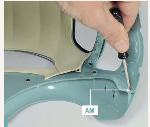
67-10. Ziehen Sie abschließend eine Schraube AM in dem auf dem Foto markierten Loch fest.
