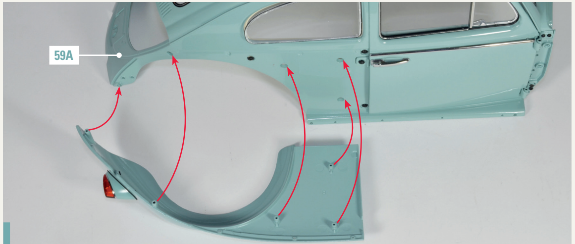
67-7. Nehmen Sie die Karosserie 59A Ihres Käfers zur Hand. Richten Sie den rechten hinteren Kotflügel wie gezeigt aus und setzen Sie ihn in die abgebildete Stelle ein.
