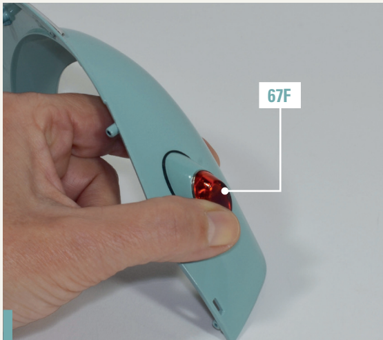
67-6. Stecken Sie die Abdeckung für die Rückleuchte 67F auf den Lampenträger, indem Sie die Teile wie auf dem Foto gezeigt ausrichten.
