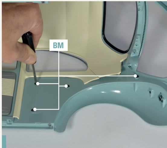
67-9. Befestigen Sie den Kotflügel, indem Sie vier Schrauben BM in den markierten Löchern festziehen.
