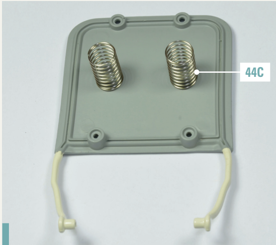
44-5. Platzieren Sie die zweite Feder 44C auf dem anderen Verbindungsstück.
