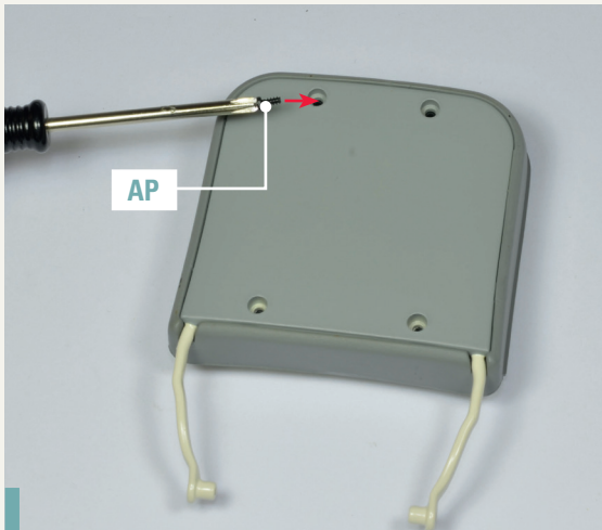
44-7. Befestigen Sie die Komponenten miteinander, indem Sie eine Schraube AP im markierten Loch festziehen.
